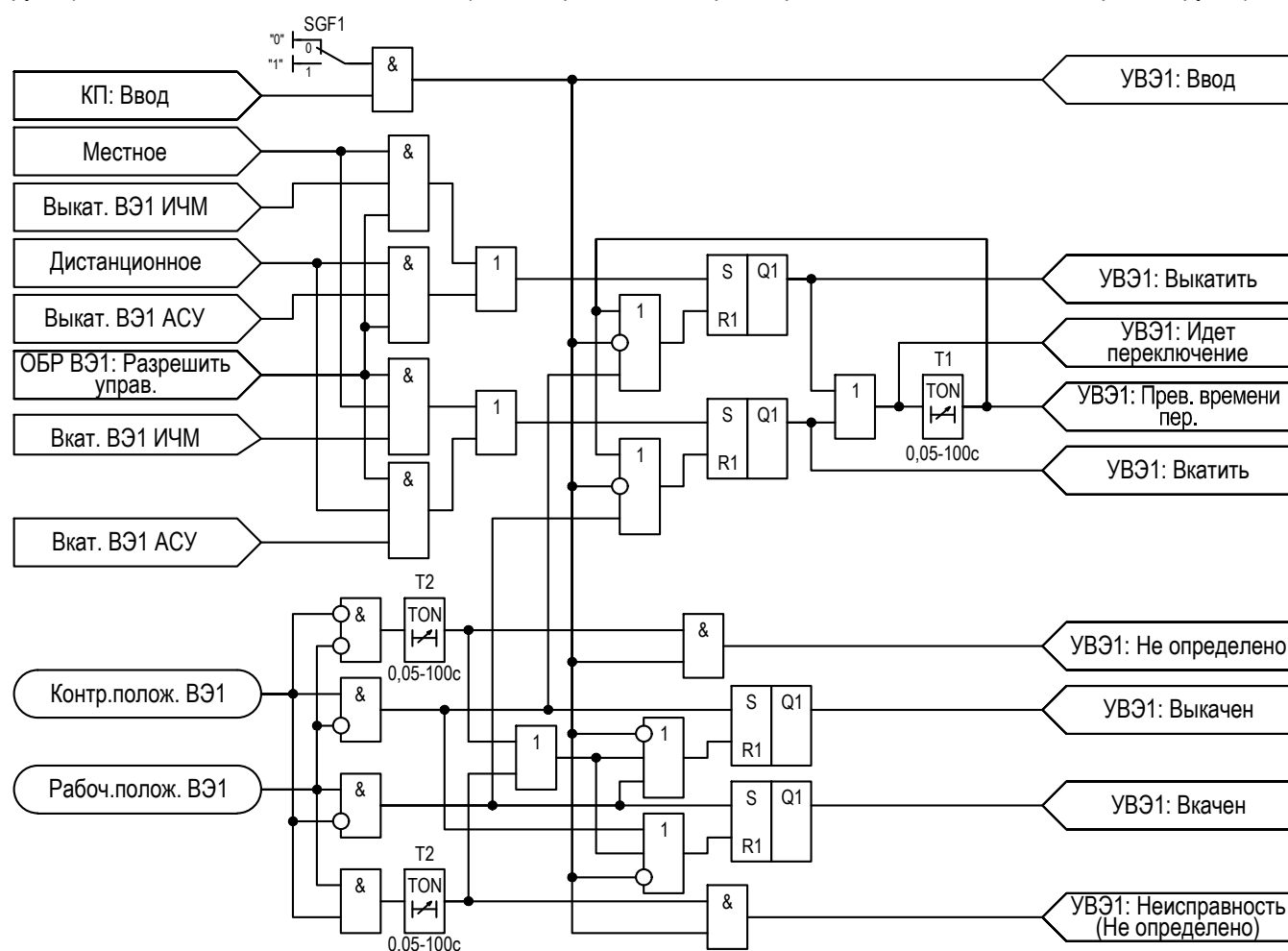
Рисунок 2.50 – Функциональная схема логики УВЭ1
