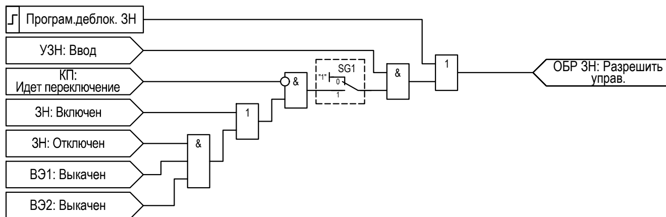
Рисунок 2.53 – Функциональная схема логики ОБР ЗН
