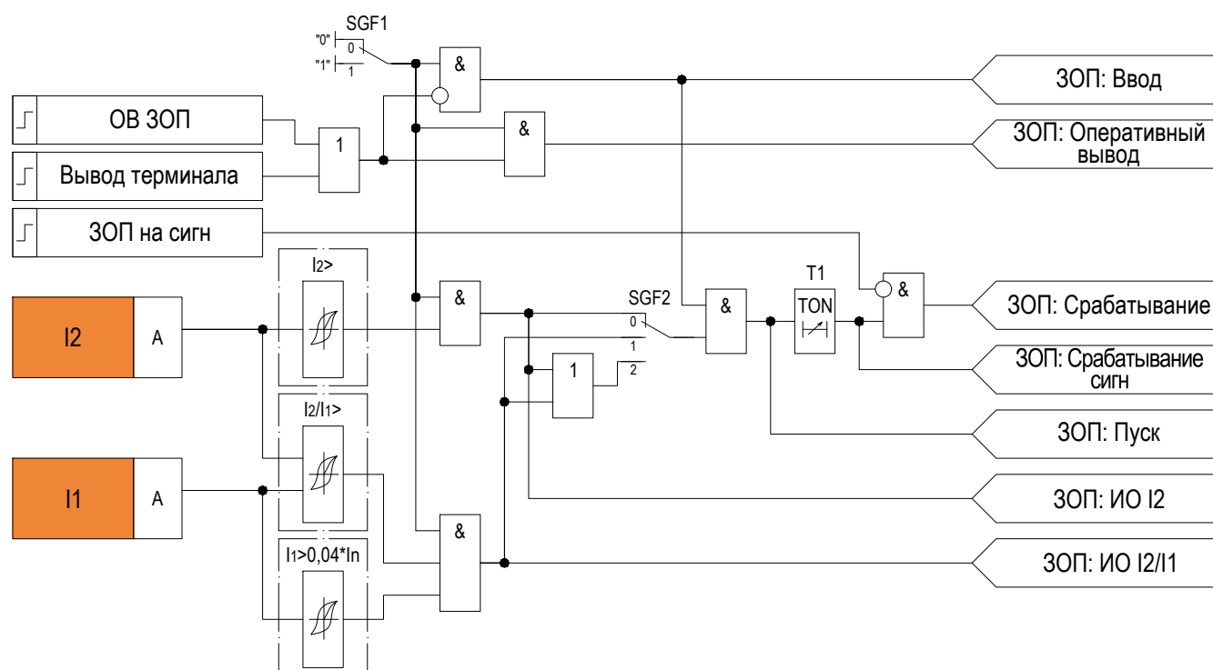
Рисунок 2.27 – Функциональная схема логики ЗОП
