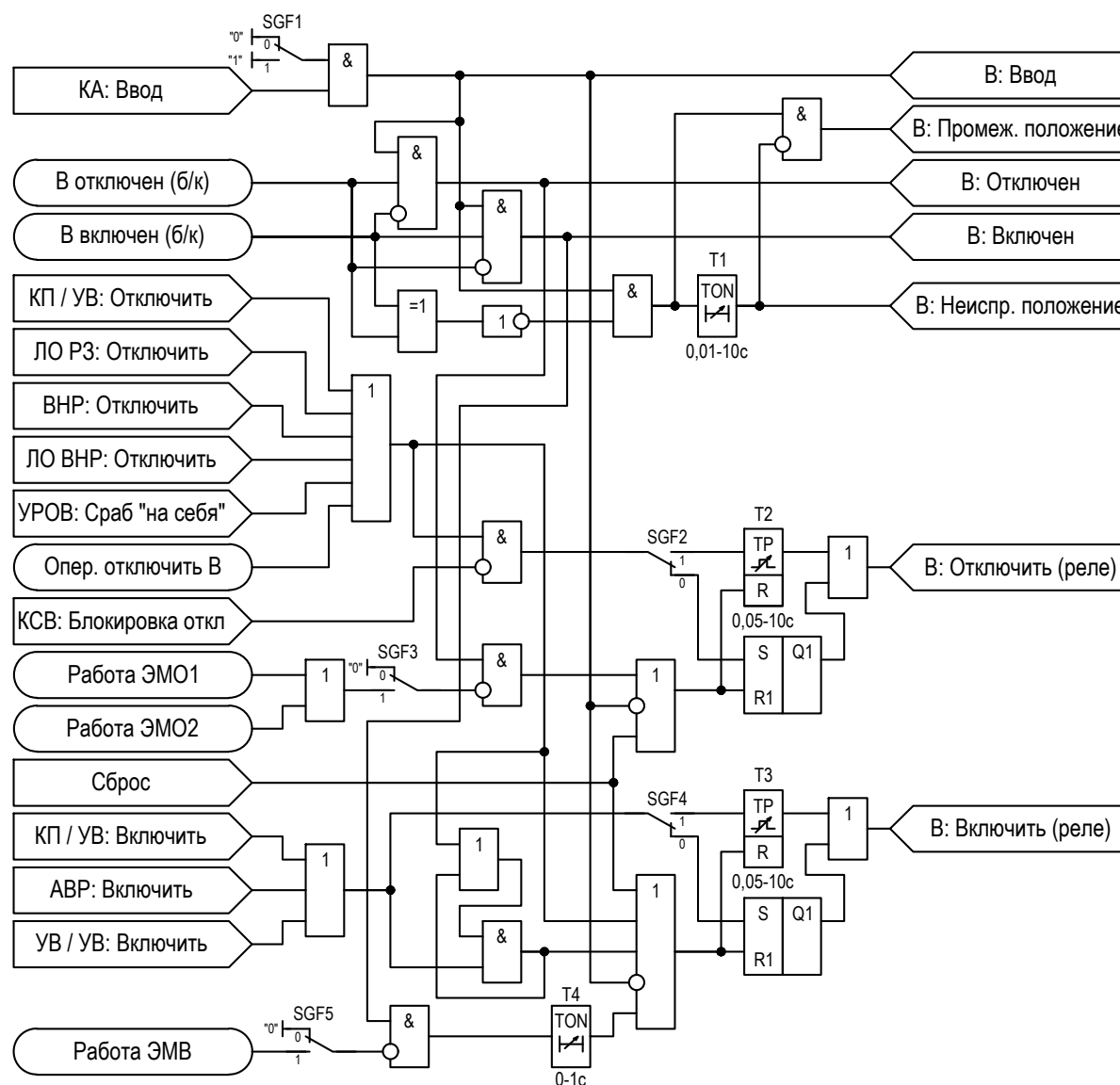
Рисунок 2.58 – Функциональная схема логики выключателя
