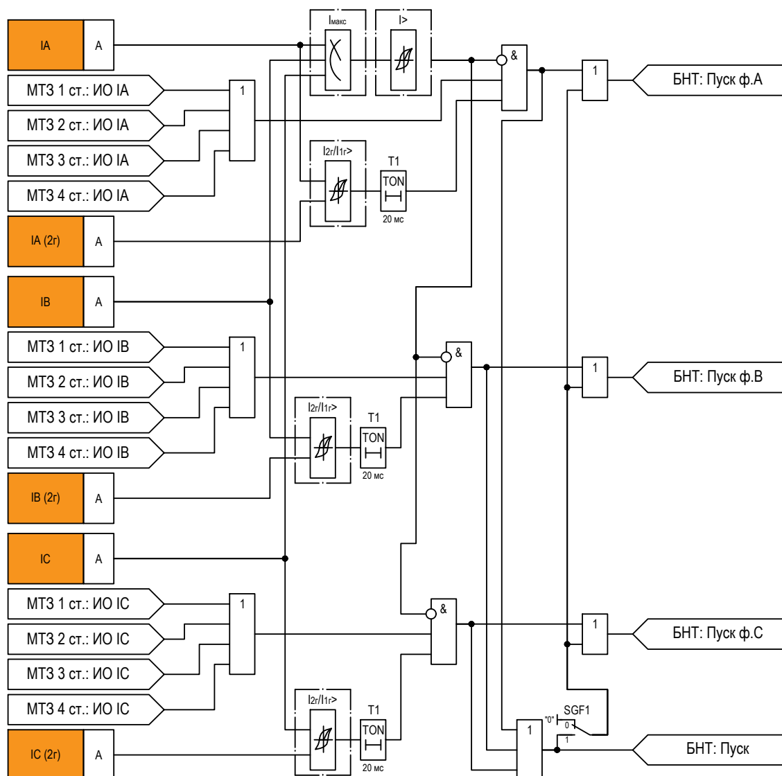
Рисунок 2.19 – Функциональная схема логики БНТ
