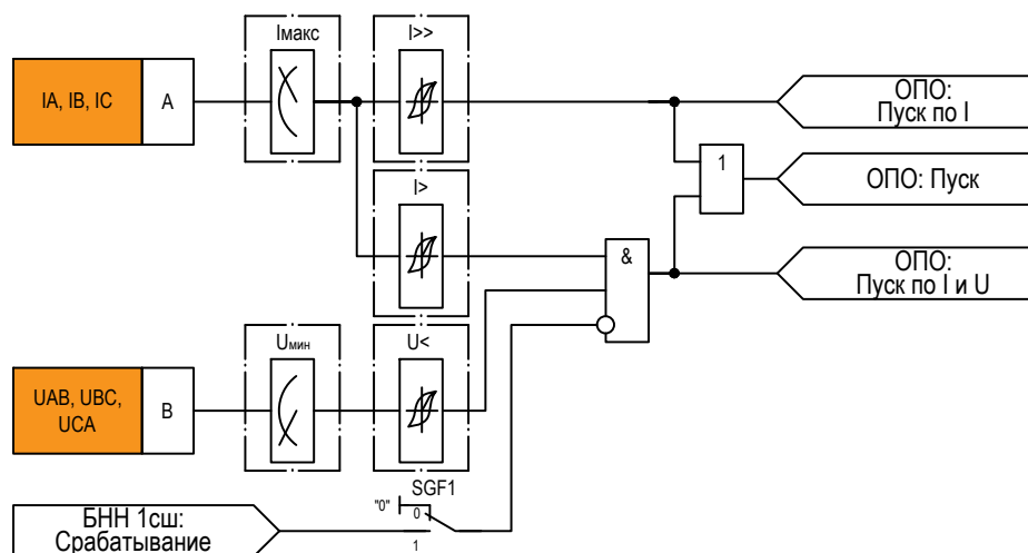
Рисунок 2.8 – Функциональная схема логики ОПО ДЗ
