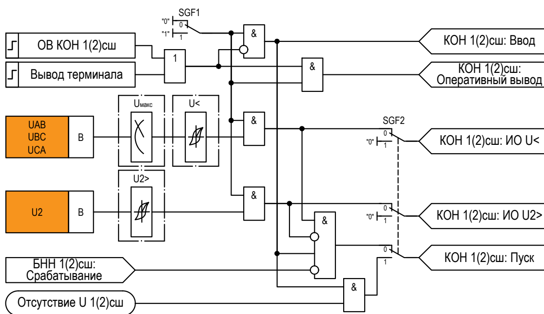
Рисунок 2.38 – Функциональная схема логики функции «КОН 1(2)сш»
