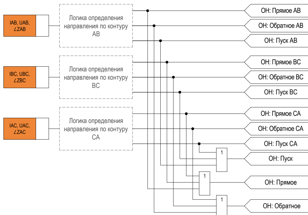
Рисунок 2.7 – Функциональная схема логики ОН
