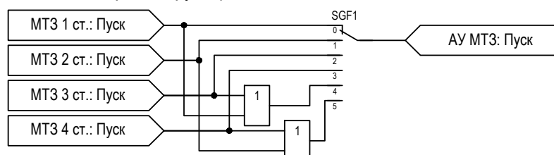
Рисунок 2.21 – Функциональная схема логики АУ МТЗ
