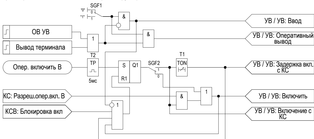
Рисунок 2.56 – Функциональная схема логики УВ
