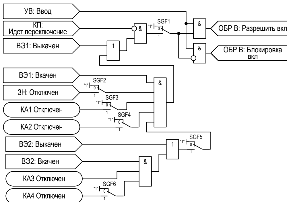
Рисунок 2.52 – Функциональная схема логики ОБР В
