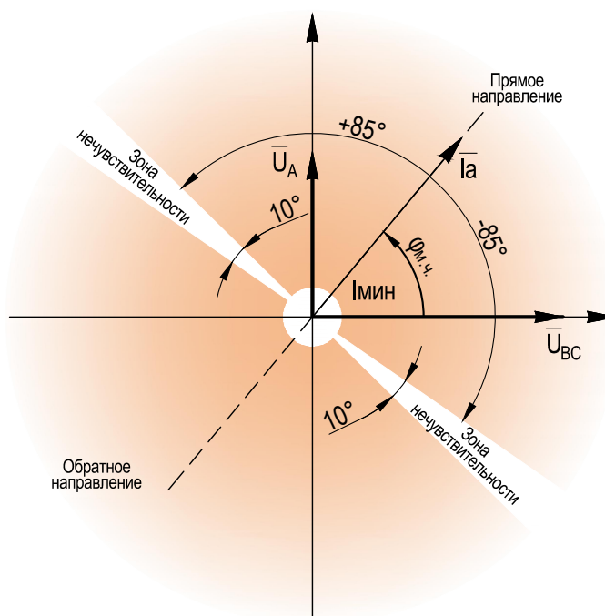
Рисунок 2.15 – Характеристика органа направления мощности
