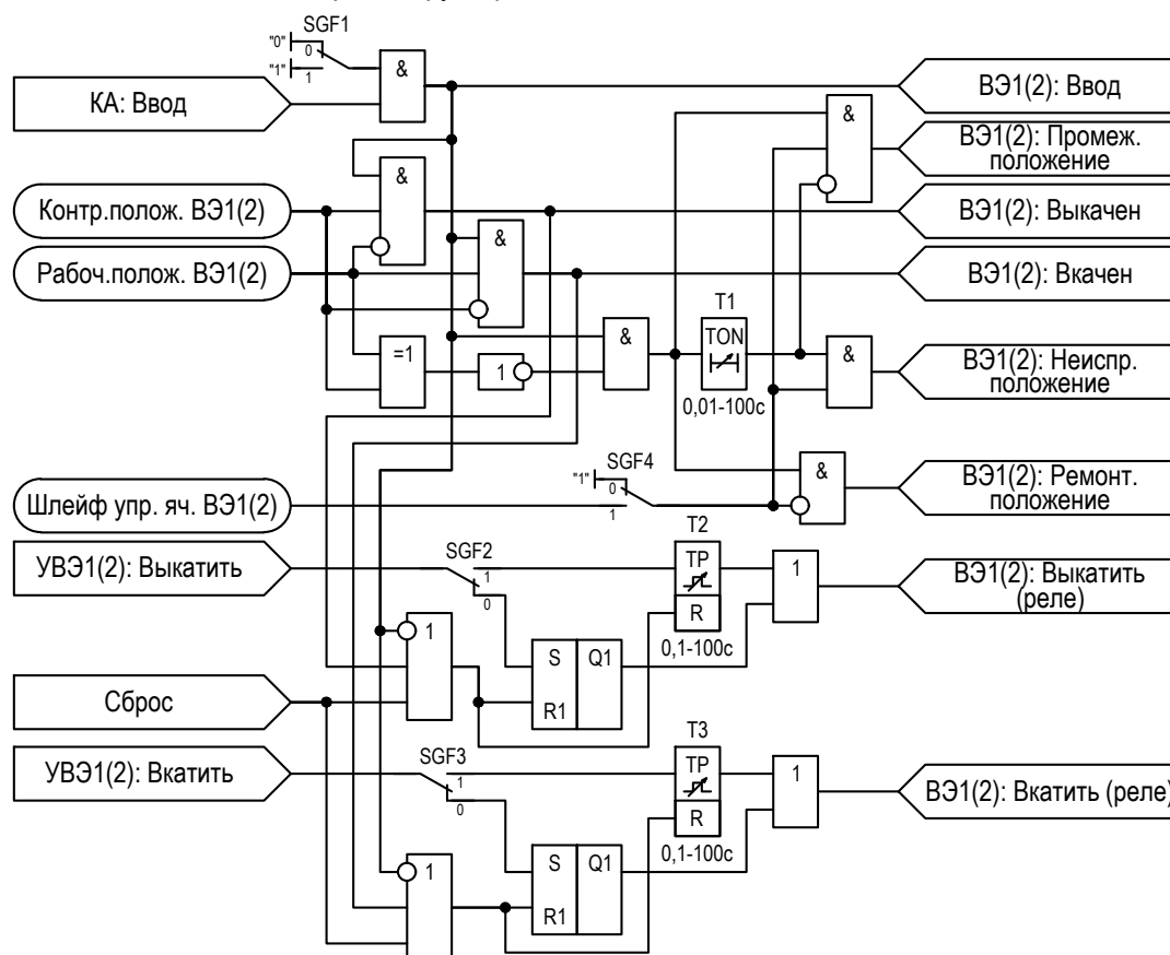
Рисунок 2.60 – Функциональная схема логики ВЭ1(2)
