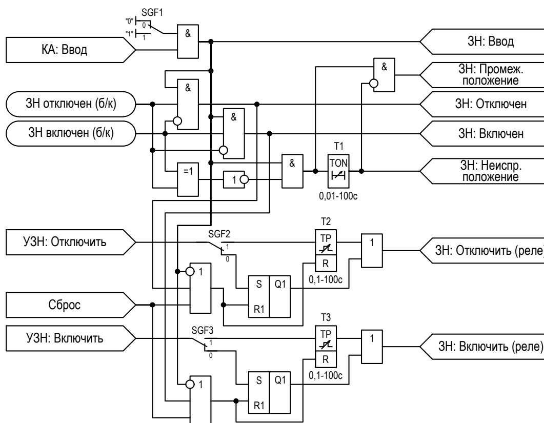
Рисунок 2.59 – Функциональная схема логики ЗН
