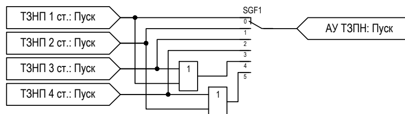
Рисунок 2.32 – Функциональная схема логики АУ ТЗНП
