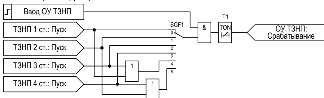
Рисунок 2.33 – Функциональная схема логики ОУ ТЗНП
