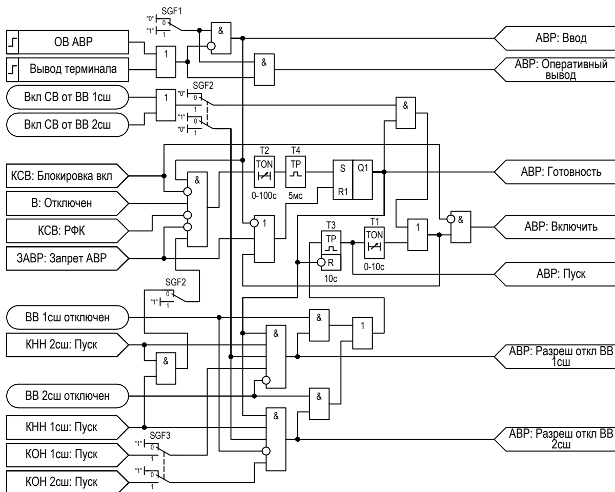
Рисунок 2.40 – Функциональная схема логики АВР
