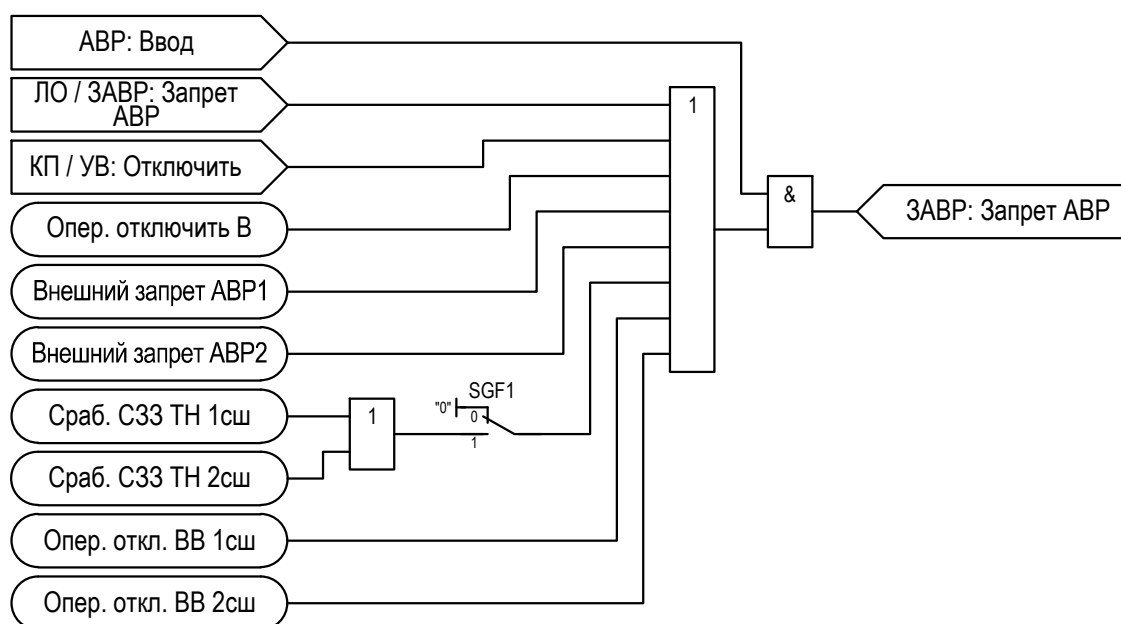
Рисунок 2.41 – Функциональная схема логики ЗАВР
