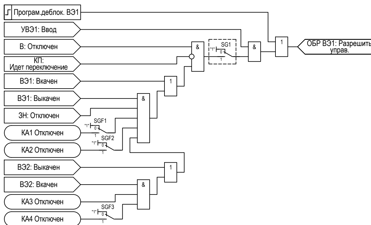
Рисунок 2.54 – Функциональная схема логики ОБР ВЭ1
