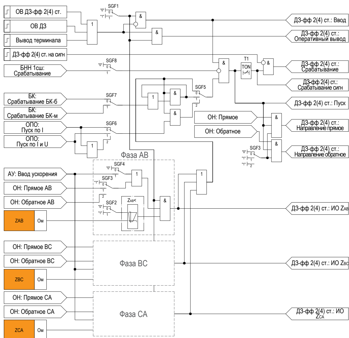
Рисунок 2.4 – Функциональная схема логики второй (четвертой) ступени ДЗ по контуру «фаза-фаза»
