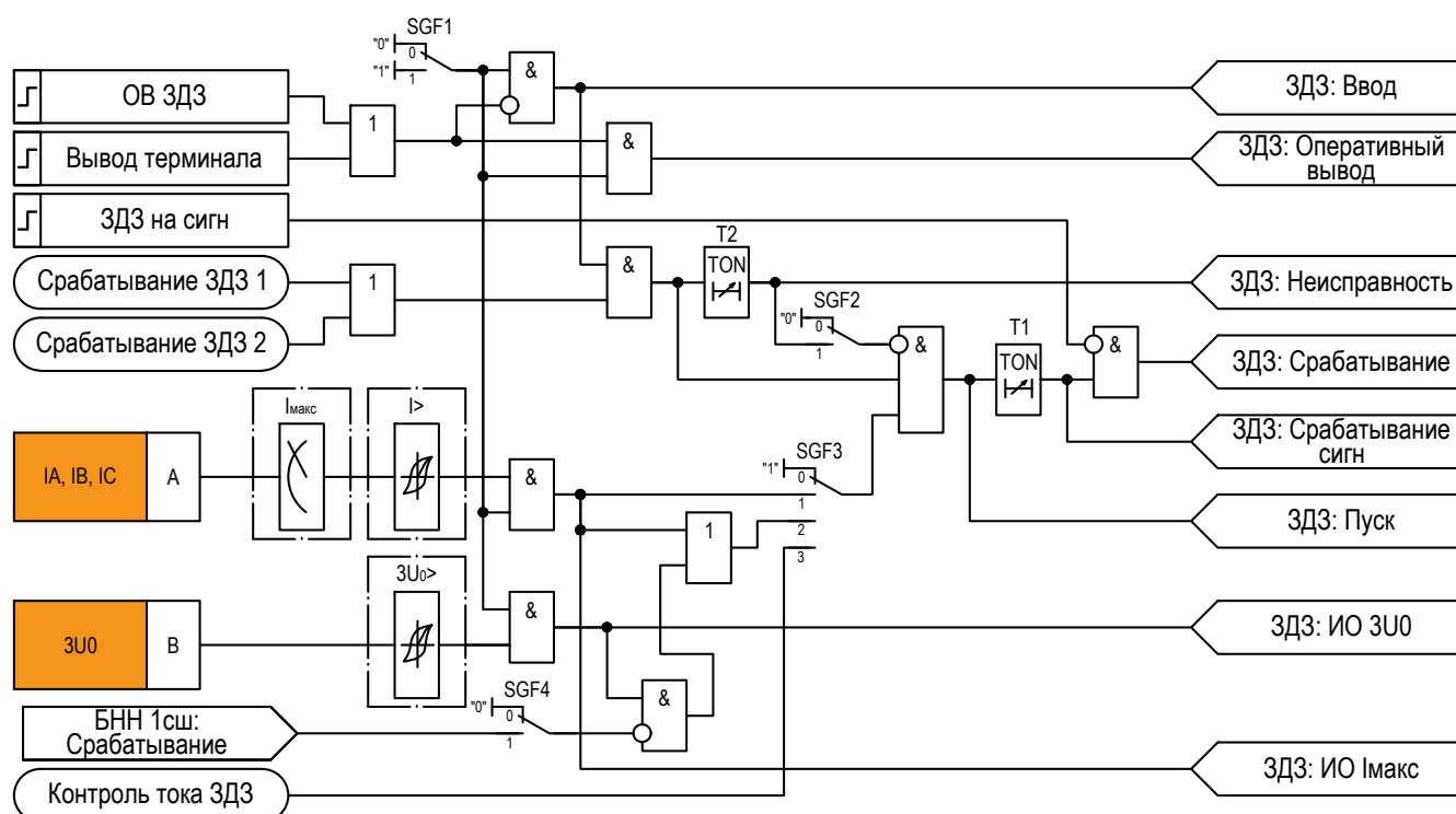
Рисунок 2.25 – Функциональная схема логики ЗДЗ
