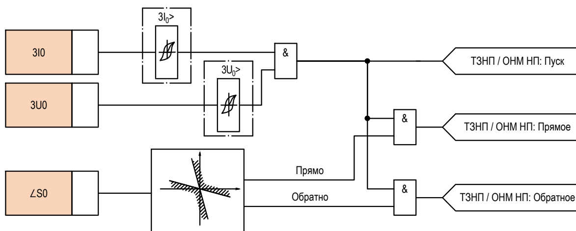
Рисунок 2.30 – Функциональная схема логики ОНМ НП
