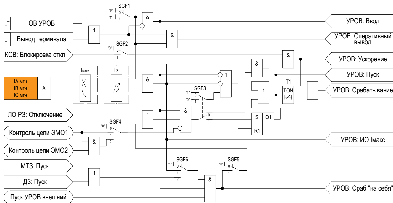
Рисунок 2.34 – Функциональная схема логики УРОВ
