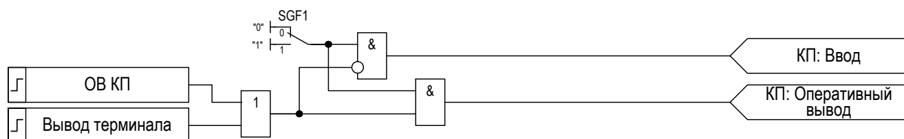
Рисунок 2.47 – Функциональная схема управления режимами работы функционального блока «КП»
