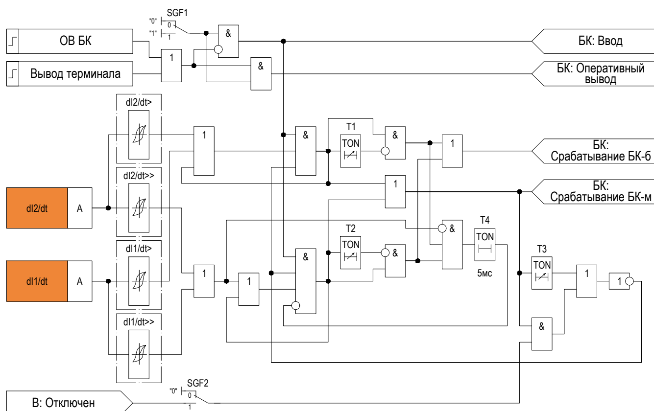
Рисунок 2.12 – Функциональная схема логики БК
