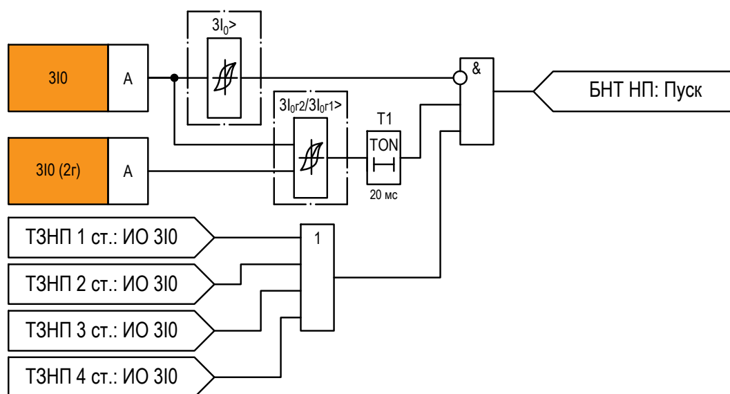
Рисунок 2.31 – Функциональная схема логики БНТ НП
