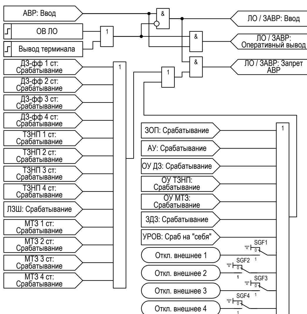
Рисунок 2.45 – Функциональная схема логики ЗАВР
