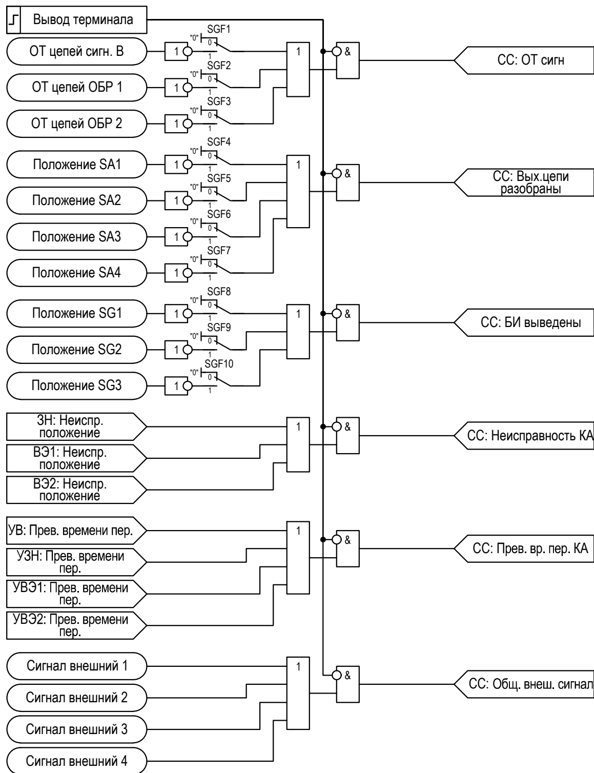
Рисунок 2.63 – Функциональная схема логики сборки сигналов
