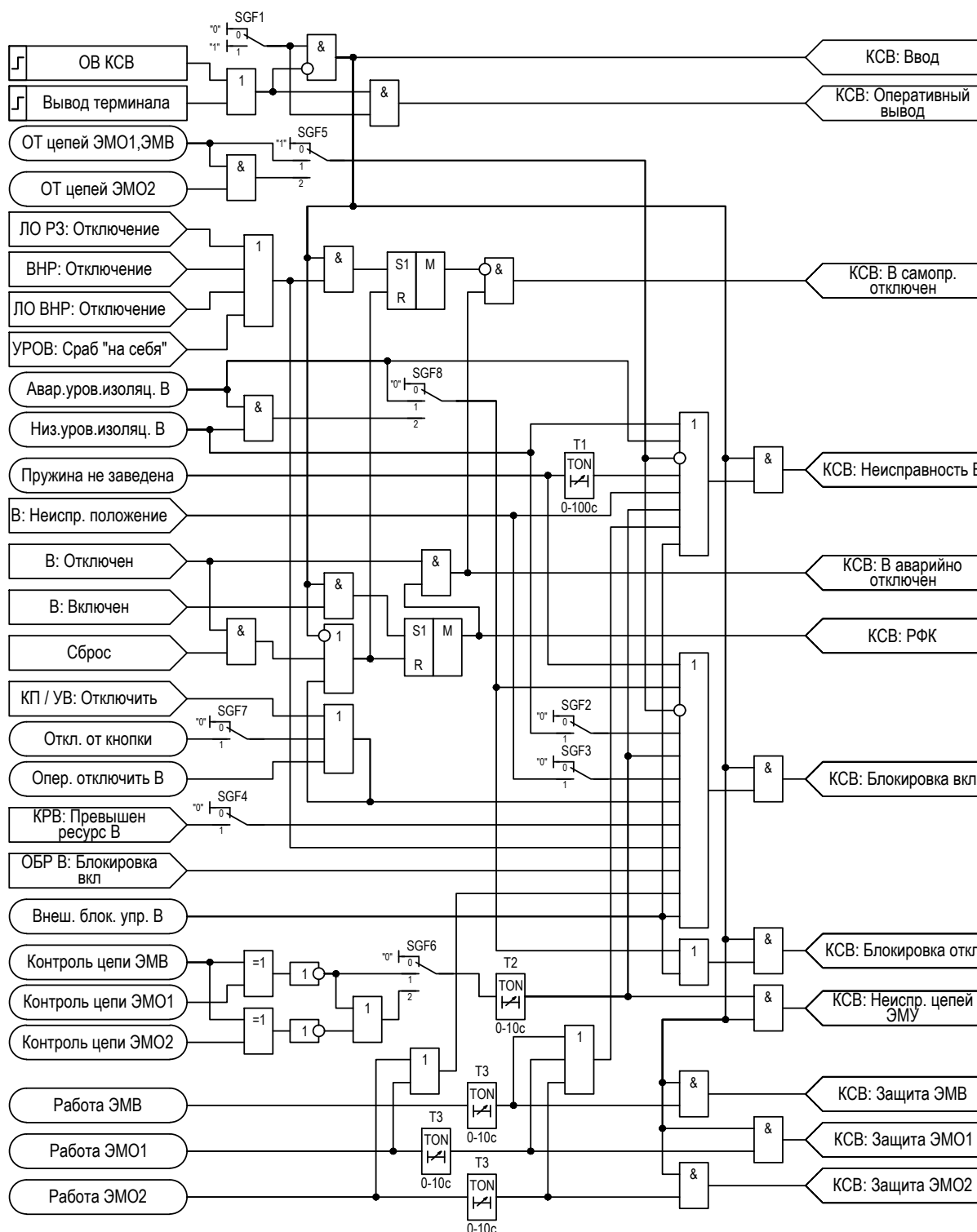
Рисунок 2.61 – Функциональная схема логики КСВ
