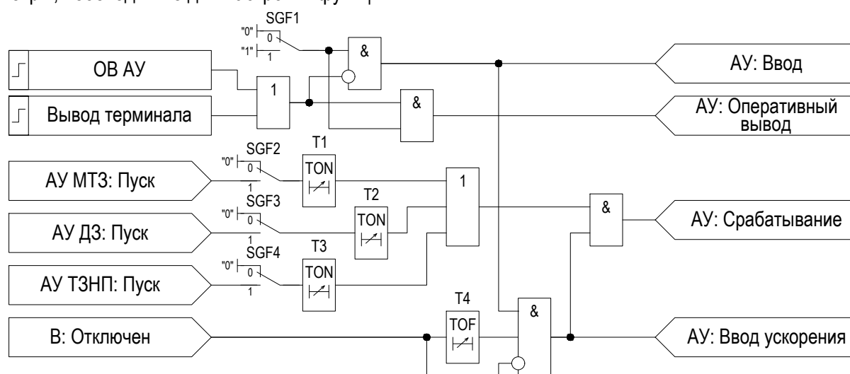
Рисунок 2.13 – Функциональная схема логики АУ
