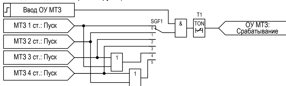
Рисунок 2.22 – Функциональная схема логики ОУ МТЗ
