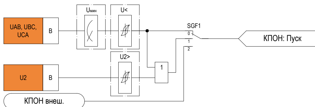
Рисунок 2.18 – Функциональная схема логики КПОН
