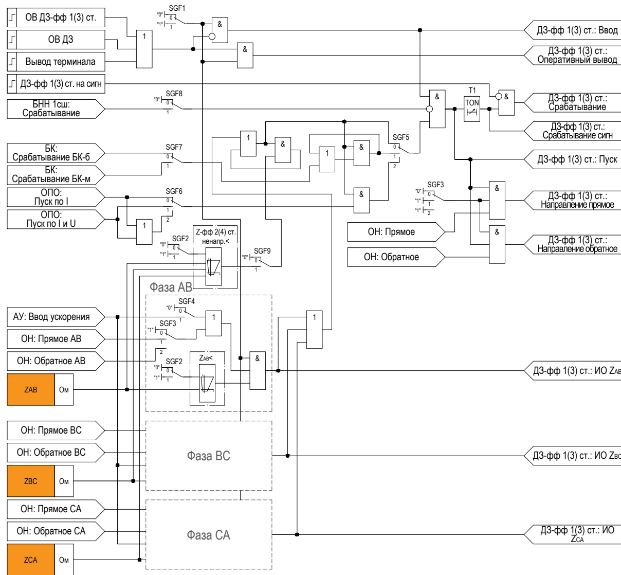
Рисунок 2.3 – Функциональная схема логики первой (третьей) ступени ДЗ по контуру «фаза-фаза»
