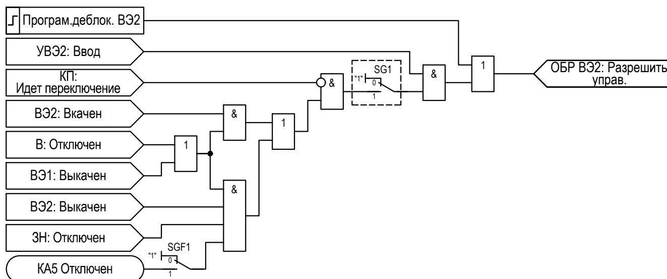
Рисунок 2.55 – Функциональная схема логики ОБР ВЭ2
