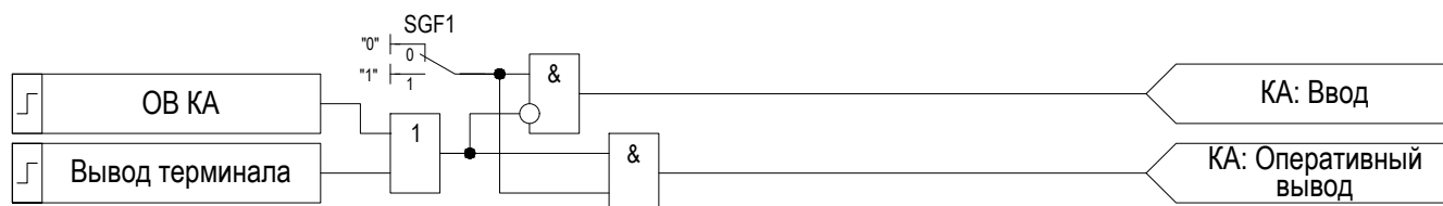
Рисунок 2.57 – Логика управления режимами КА
