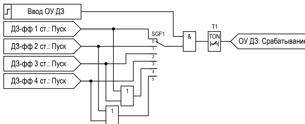
Рисунок 2.10 – Функциональная схема логики ОУ ДЗ
